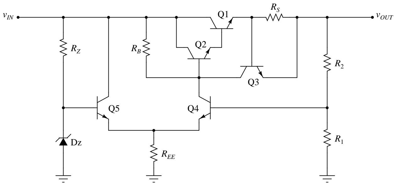
Slika 1: Stabilizator napona sa diskretnim komponentama.
